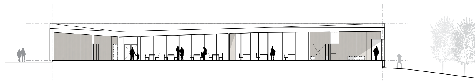
snitt BB_mot kirken 1:200
